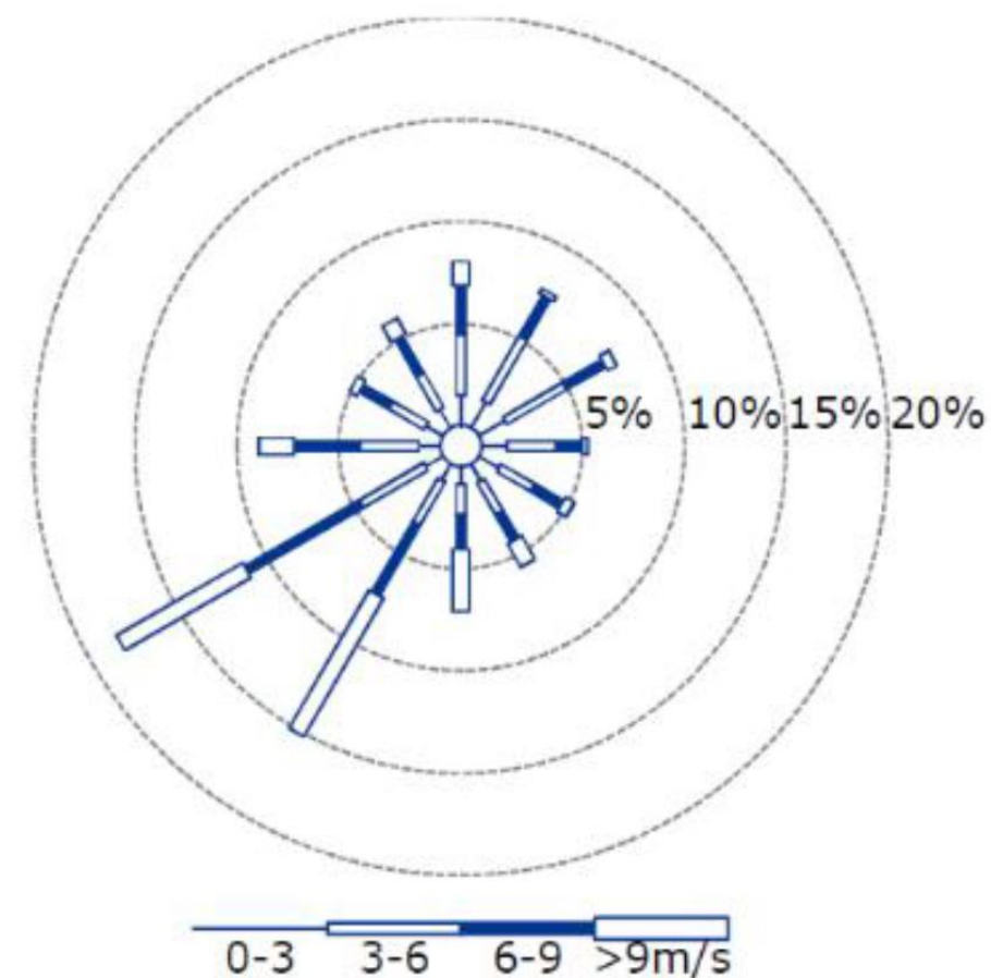
Figure 7 : Rose des vents (source : Orféa Acoustique, 2018)
